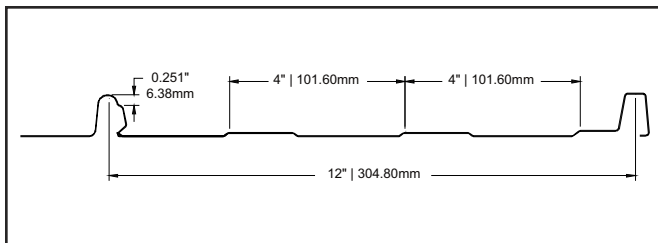
SNAP LOK 12"
