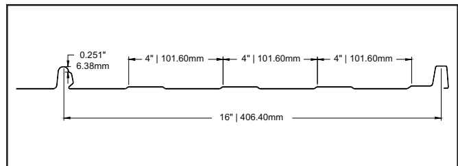
SNAP LOK 16"
